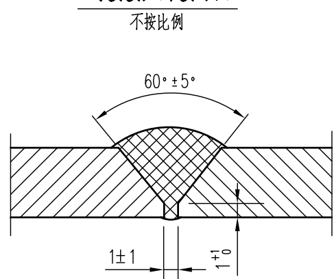
对接接头焊接详图
