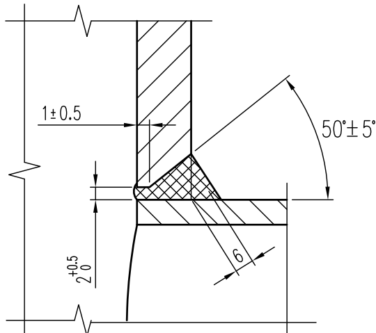
非径向齐平接管焊接详图
