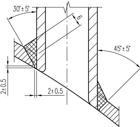
非径向齐平接管焊接详图
